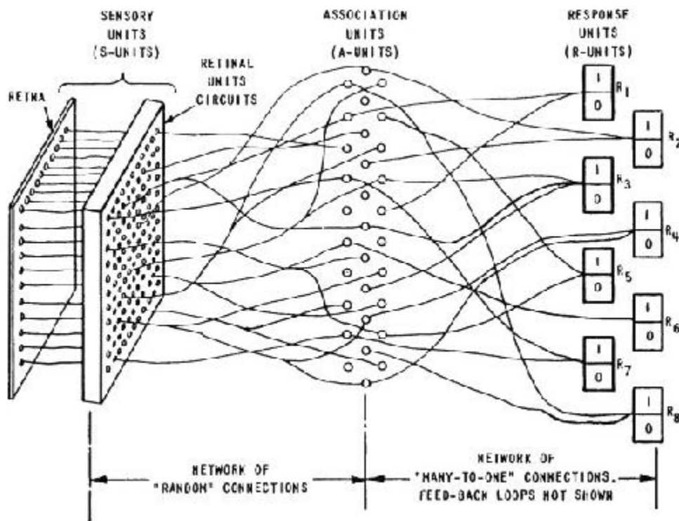
感知机的示意图
